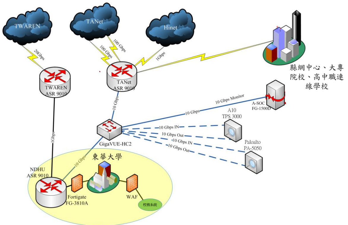
花蓮區網中心資安防護網路架構圖（2018Q4）
