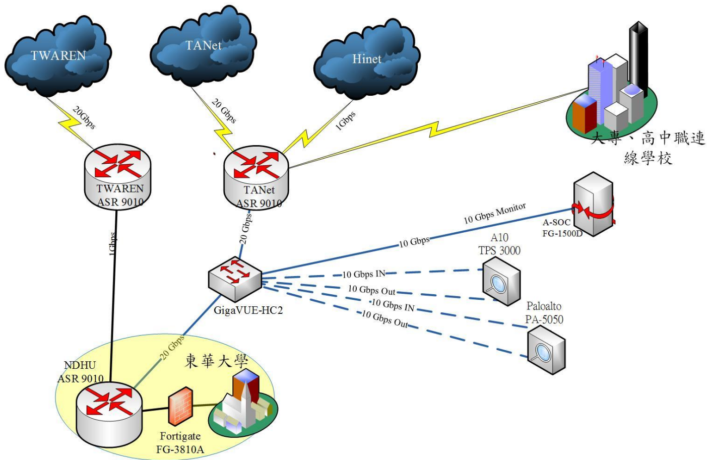
花蓮區網中心資安防護網路架構圖（2017Q4）
